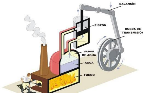
Esquema d'una màquina de vapor
